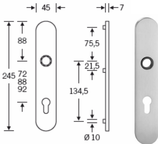
Escutcheon #12.222.508Z
