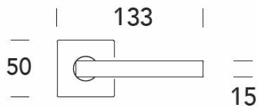
LEVER 14.J3733 Jado
